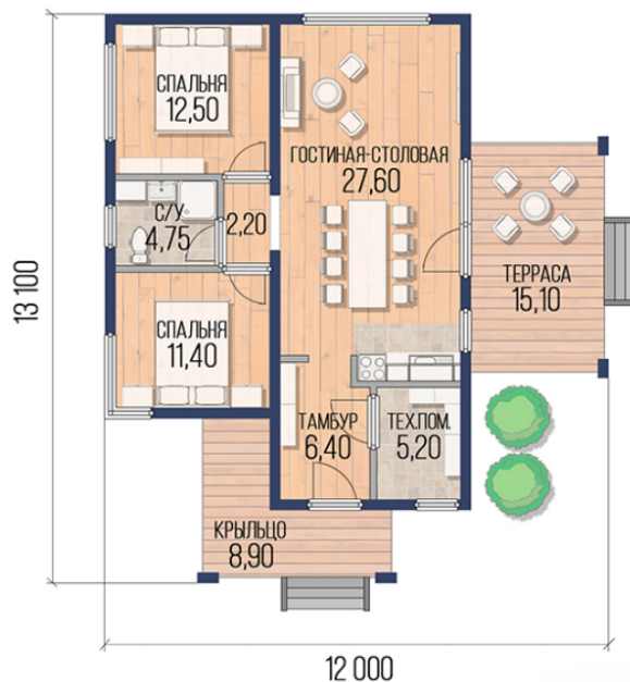
ПЛАН ПОМЕЩЕНИЯ 75,65 м 2
